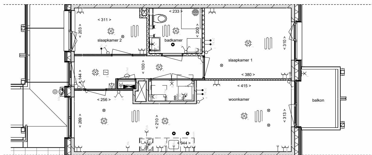
plattegrond
